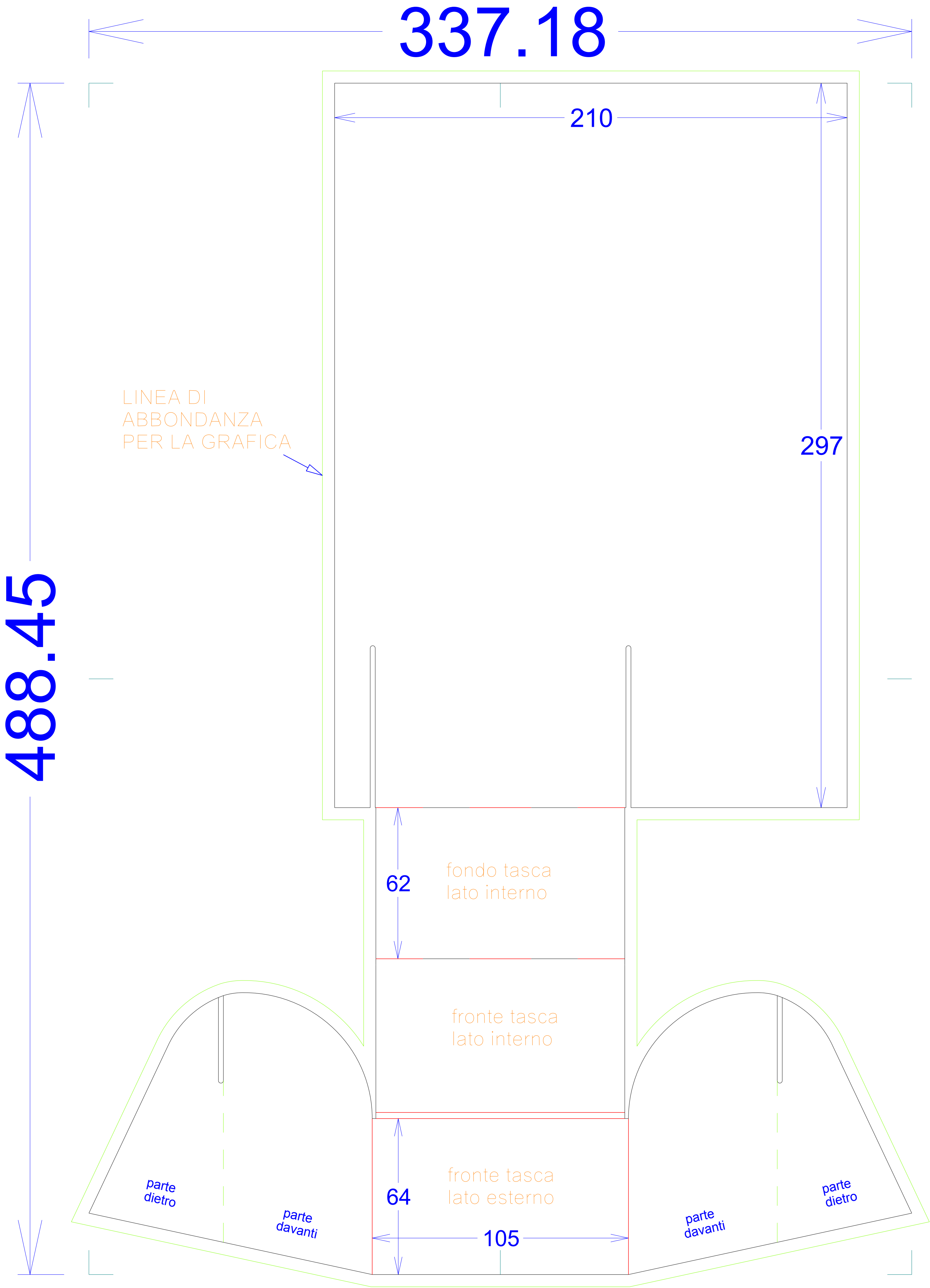
PINZA LATO STAMPA COD.800_3001-01_DIS1
